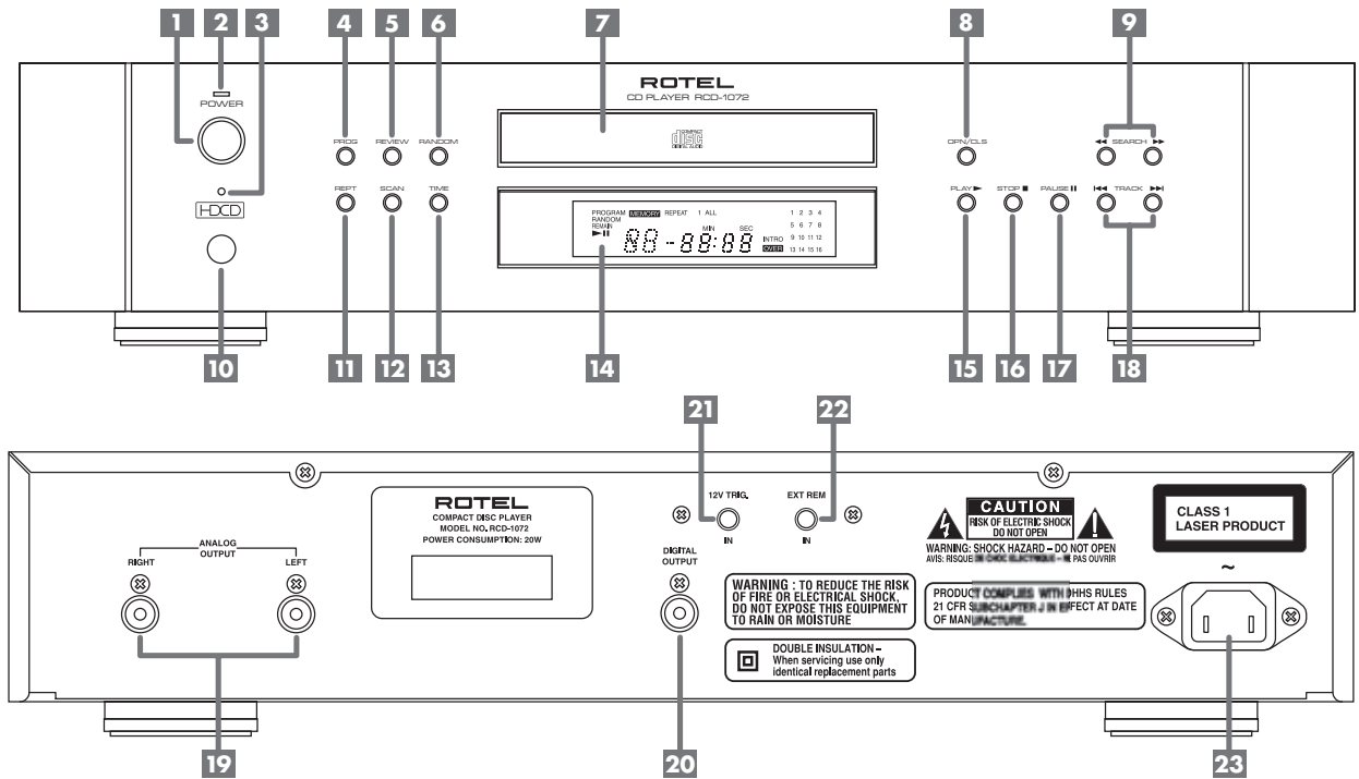
Figure 1: Controls and Connections Commandes et branchements Bedienelemente und Anschlüsse Controlli e collegamenti Controlos y Conexiones Bedieningsorganen en aansluitingen Funktioner och anslutningar
